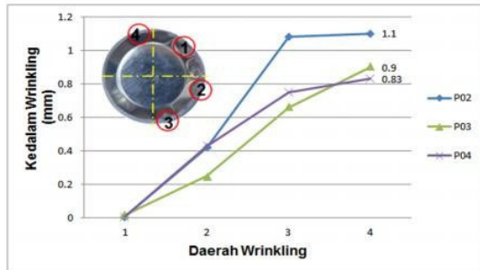
Gambar 15. Grafik Distribusi Cacat ( Wrinkling ) Setiap Blank Dengan Pelumasan Dengan BHF 2,352 Nm Per Baut
