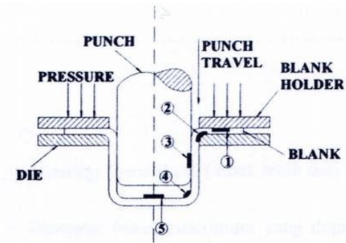
Gambar 2. Tahap proses deep drawing untuk cylinder cup
