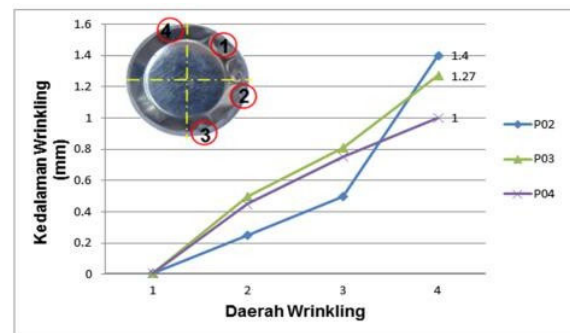
Gambar 13. Grafik Distribusi Cacat (Wrinkling) Setiap Blank Tanpa Pelumasan Dengan BHF 1,7652 Nm Per
