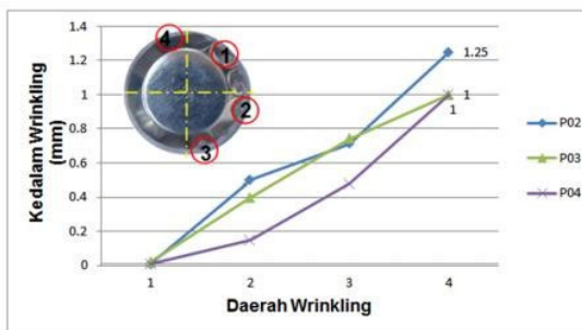
Gambar 16. Grafik Distribusi Cacat ( Wrinkling ) Setiap Blank Dengan Pelumasan Dengan BHF 1,7652 Nm Per Baut
