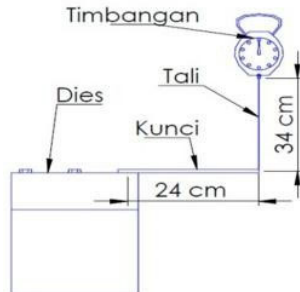
Gambar 10. Kunci Momen Modifikasi
