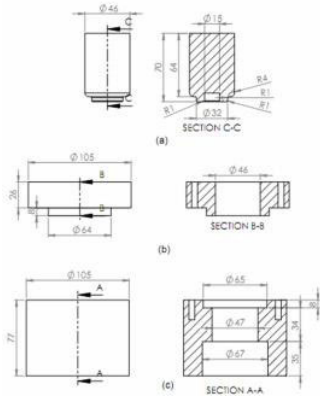
Gambar 8. (a) Desain Punch (b) Desain Blank Holder (c) Desain Dies
