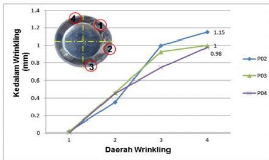
Gambar 15. Grafik Distribusi Cacat ( Wrinkling ) Setiap Blank Dengan Pelumasan Dengan BHF 2,352 Nm Per Baut
