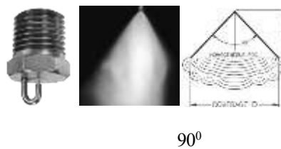
Gambar 4. Karakteristik semprotan nosel PJ32
