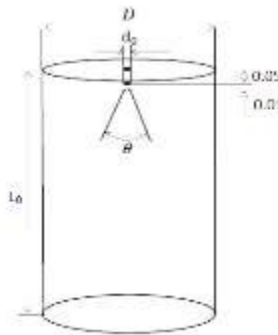
Gambar 2. Geometri Cerobong dan Nosel
