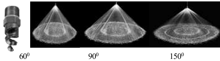
Gambar 3. Karakteristik semprotan nosel TF6
