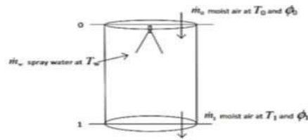
Gambar 4.11 Sistem Aliran Massa Pada Cerobong Evaporasi (Sarjito, 2012)
