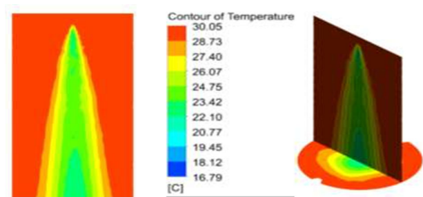
Gambar 8. Kontur temperatur hasil simulasi jenis Rossin rammler
