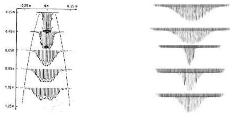
Gambar 7. Profil kecepatan
